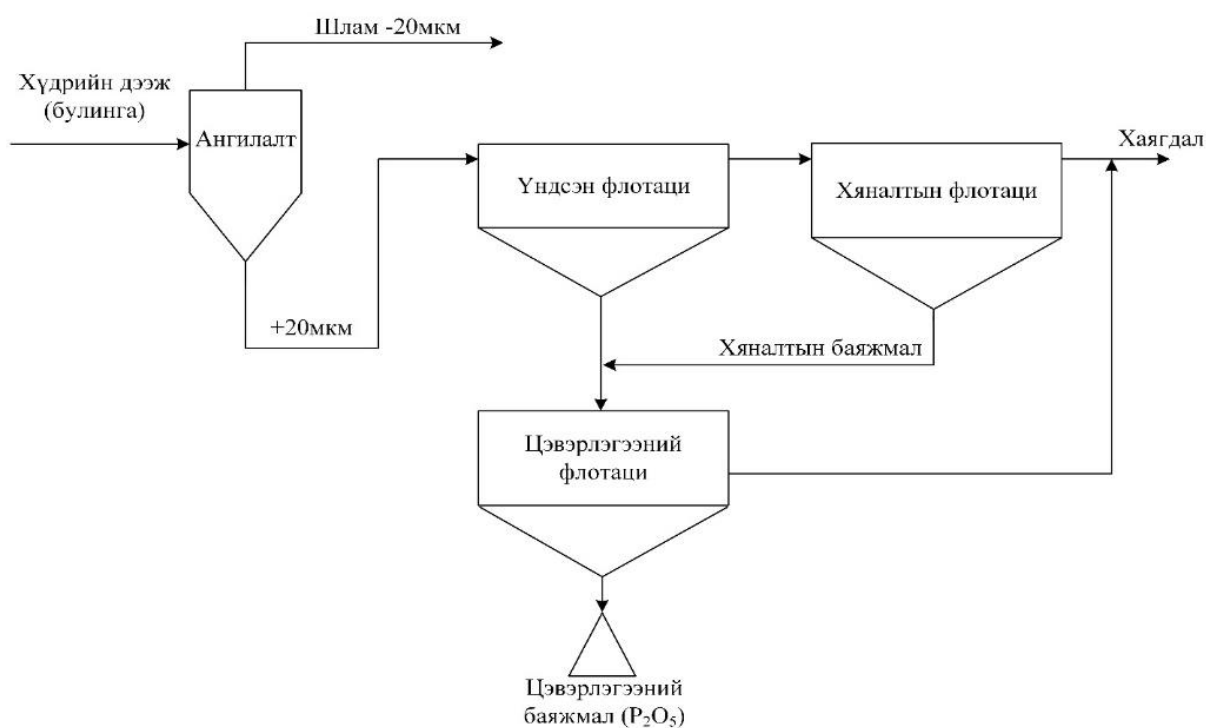
Хавсралт зураг 1. Флотацийн нэг шатны цэвэрлэгээ бүхий туршилтын схем
