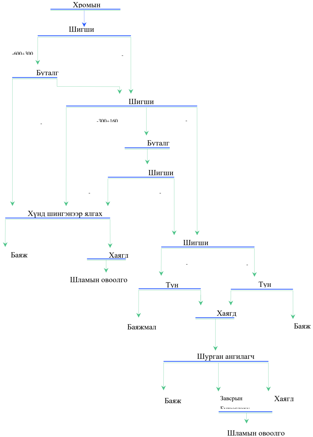
Зураг-1. Донскийн УБҮ-ийн гравитацийн баяжуулалтын технологийн схем
